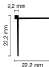
TEL 20: Eckleiste (Außenecke) für saubere Tapetenabschlüsse
