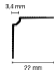
TIW 20: Innenwinkel für saubere Tapetenabschlüsse
